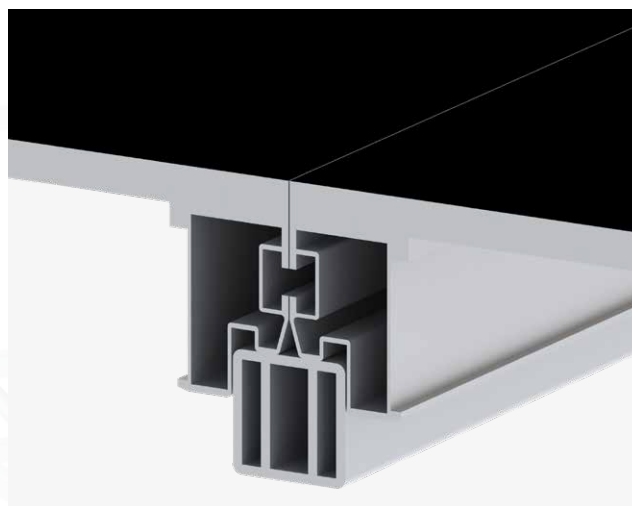
поперечное сечение
